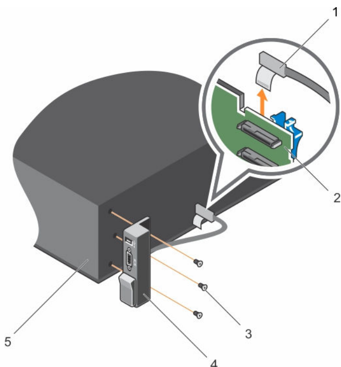
Figure 59. Retrait et installation du panneau du I/O
