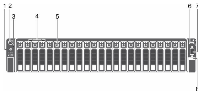
Figure 1. Châssis de disque dur ou SSD de 2,5 pouces
