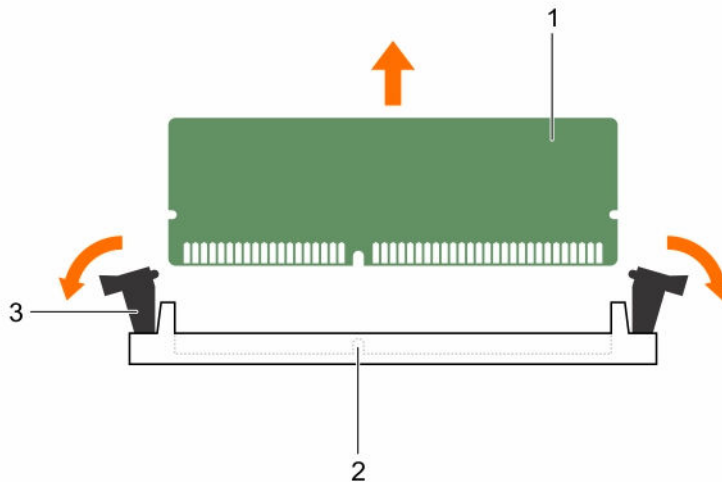
Figure 18. Retrait et installation d'une barrette de mémoire
