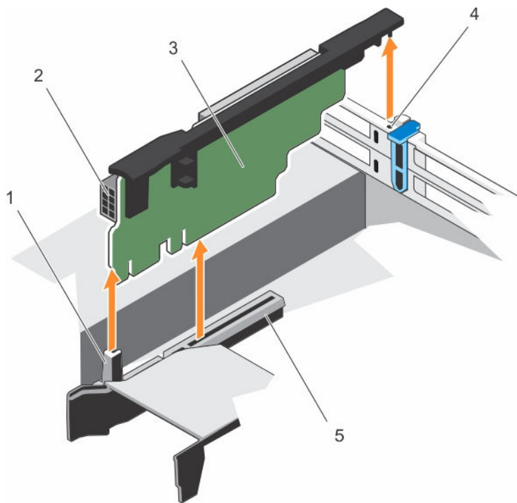
Figure 37. Retrait et installation de la carte de montage pour carte d'extension 3
