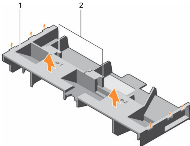
Figure 13. Retrait et installation du carénage de refroidissement
