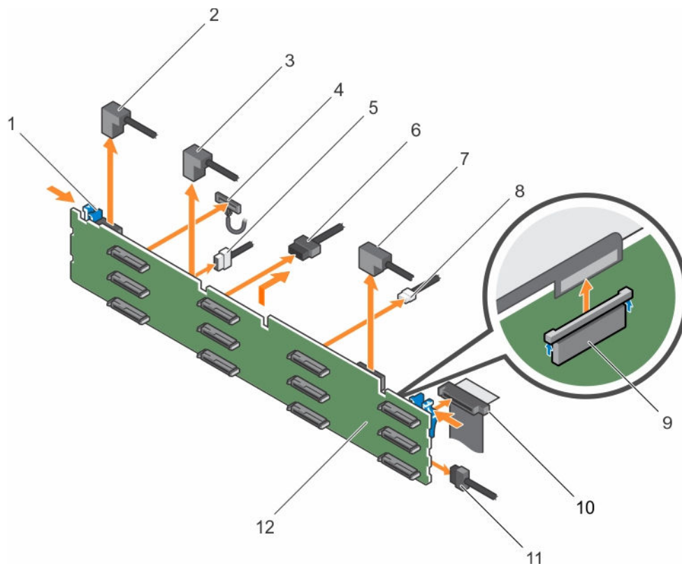
Figure 56. Retrait et installation du fond de panier SAS/SATA de 3,5 pouces (x12)
