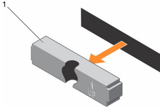
Figure 50. Retrait et installation d'un cache de disque dur de 2,5 pouces (arrière)
