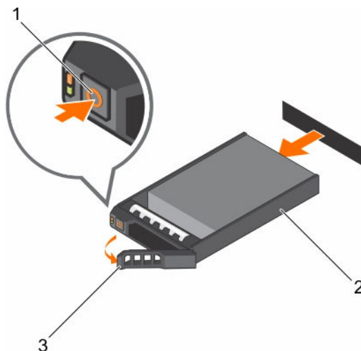
Figure 52. Retrait et installation d'un disque dur remplaçable à chaud
