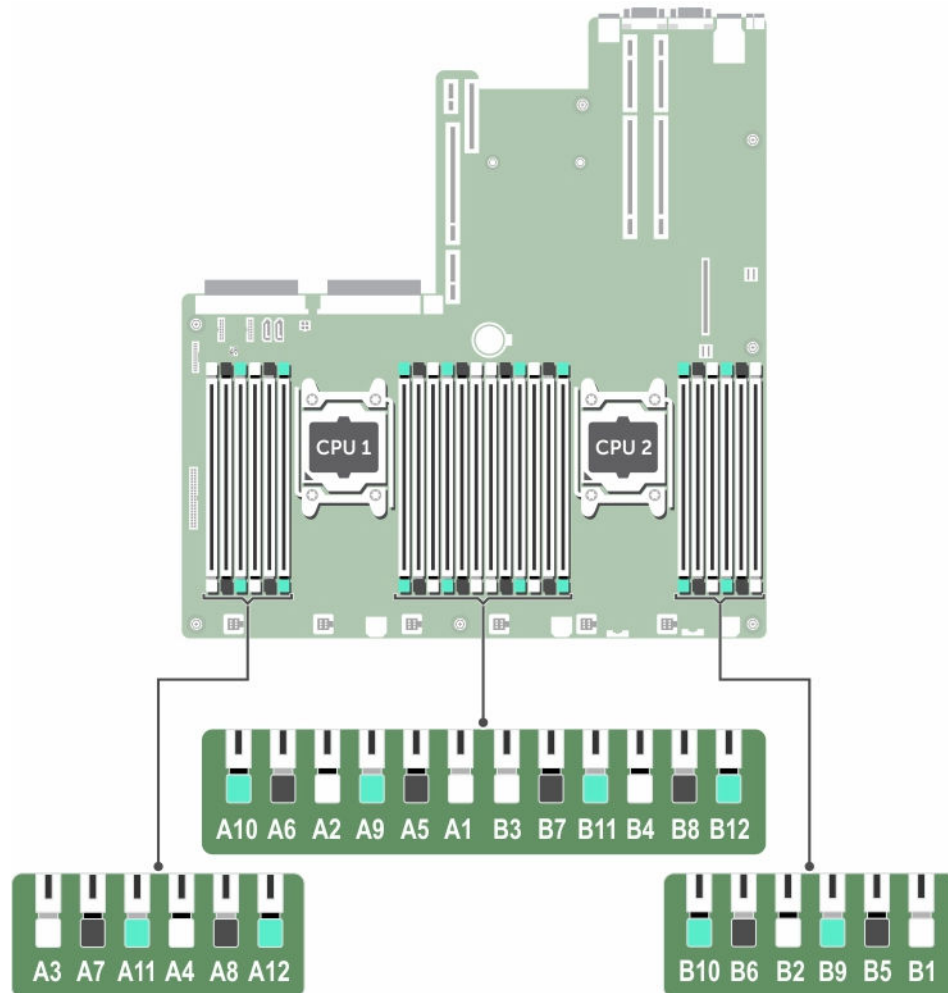
Figure 17. Emplacement des supports de mémoire
