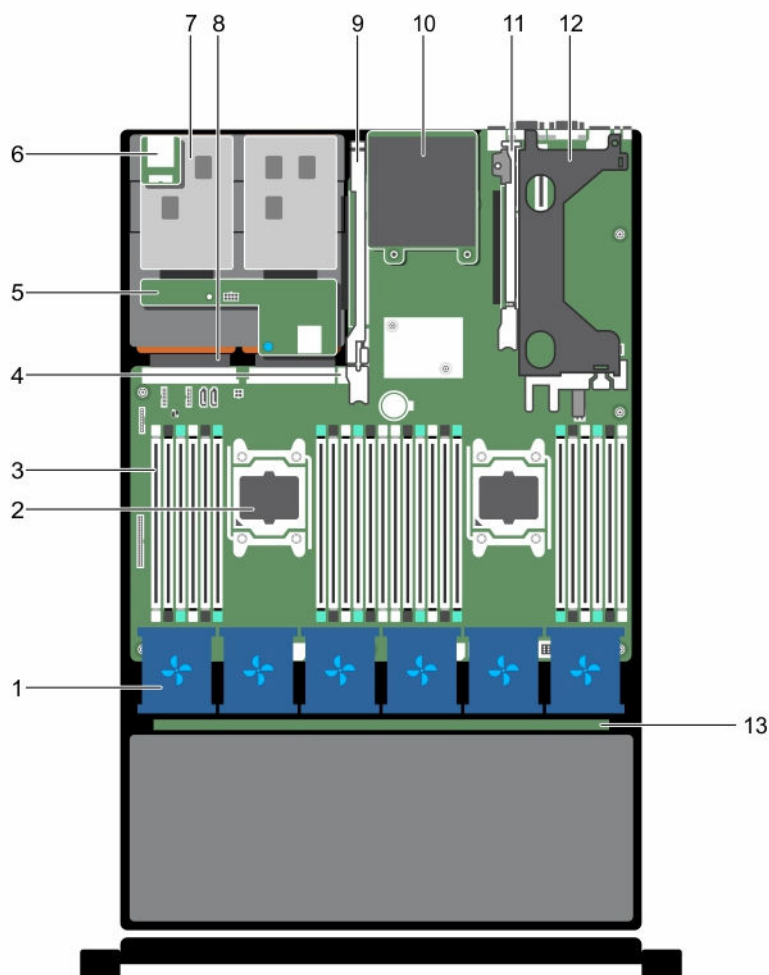
Figure 12. À l'intérieur du système : Dell XC730xd
