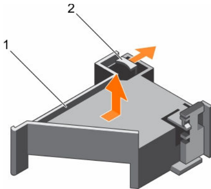
Figure 27. Retrait et installation du support de carte PCIe
