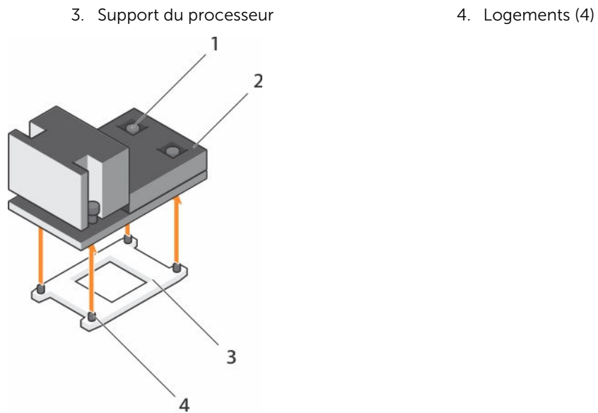
Figure 22. Retrait et installation du dissipateur de chaleur du processeur
