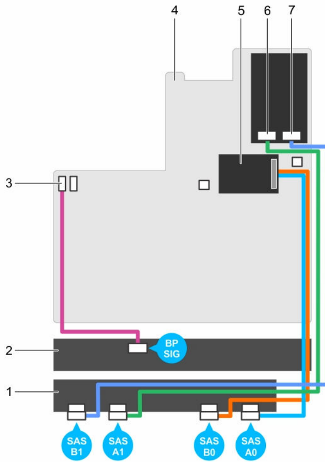
Figure 55. Schéma de câblage : fond de panier SAS/SATA de 2,5 pouces (x24) (option 2)
