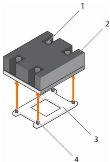
Figure 23. Retrait et installation du dissipateur de chaleur du processeur
