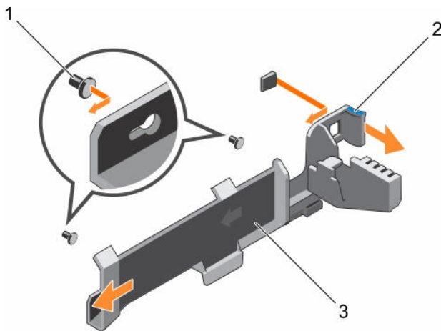
Figure 29. Retrait et installation du support de fixation des câbles
