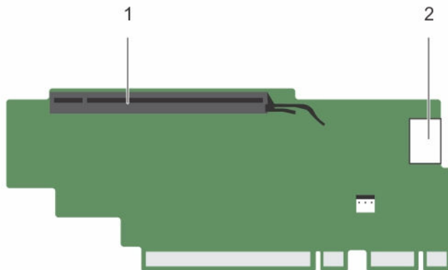
Figure 39. Identification des connecteurs de la carte de montage pour carte d'extension 3 (alternative).
