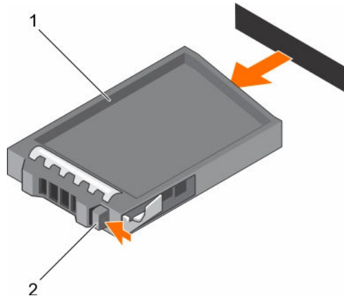
Figure 49. Retrait et installation d'un cache de disque dur de 2,5 pouces
