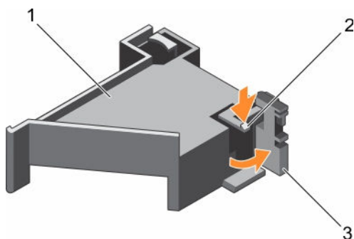
Figure 28. Ouverture et fermeture du loquet du support de carte PCIe
