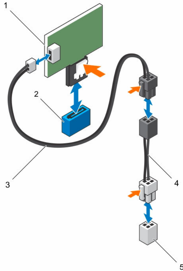
Figure 20. Retrait et installation du SATADOM
