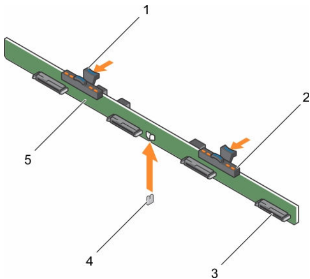
Figure 60. Retrait et installation du fond de panier de disque dur de 3,5 pouces (x4)
