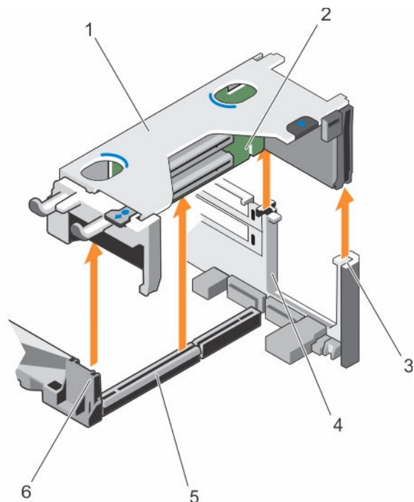
Figure 33. Retrait et installation de la carte de montage pour carte d'extension 1
