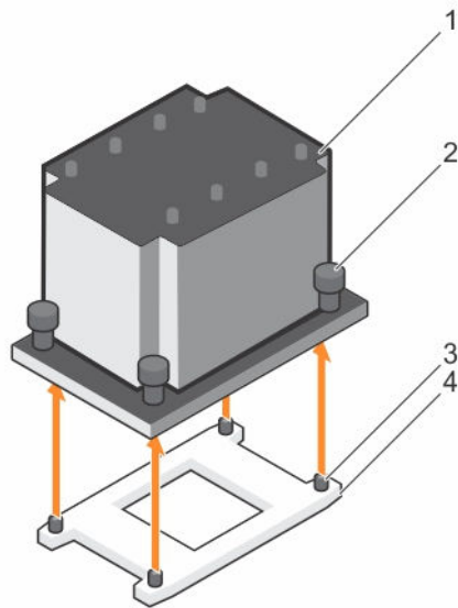
Figure 21. Retrait et installation d'un processeur
